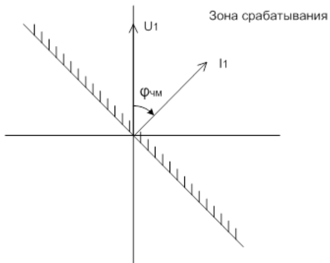
Рисунок 13 – Характеристика срабатывания РНМ МТЗ НН1 (НН2, НН3)
