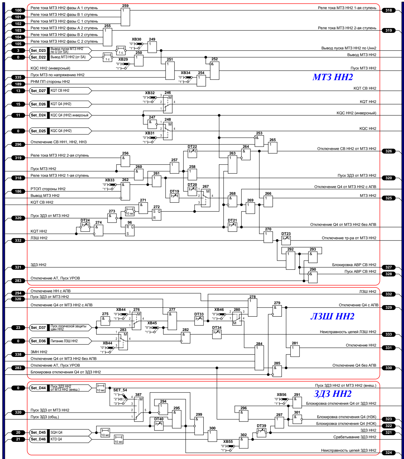
Рисунок 9 – Функциональная логическая схема блока логики МТЗ НН2, ЛЗШ НН2, ЗДЗ НН2
