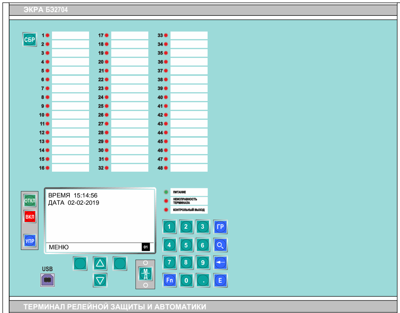
Рисунок 16 – Расположение элементов на передней панели терминала защиты БЭ2704 308 (лицевая панель терминала с 48 светодиодами)
