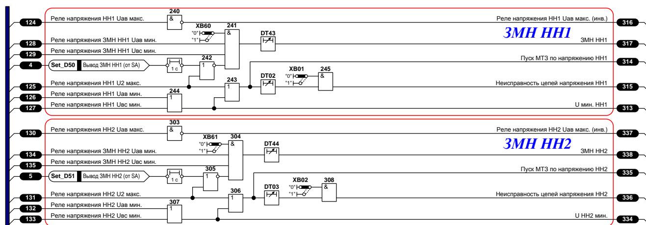
Рисунок 5 – Функциональная логическая схема блока логики ЗМН НН1 (НН2, НН3)
