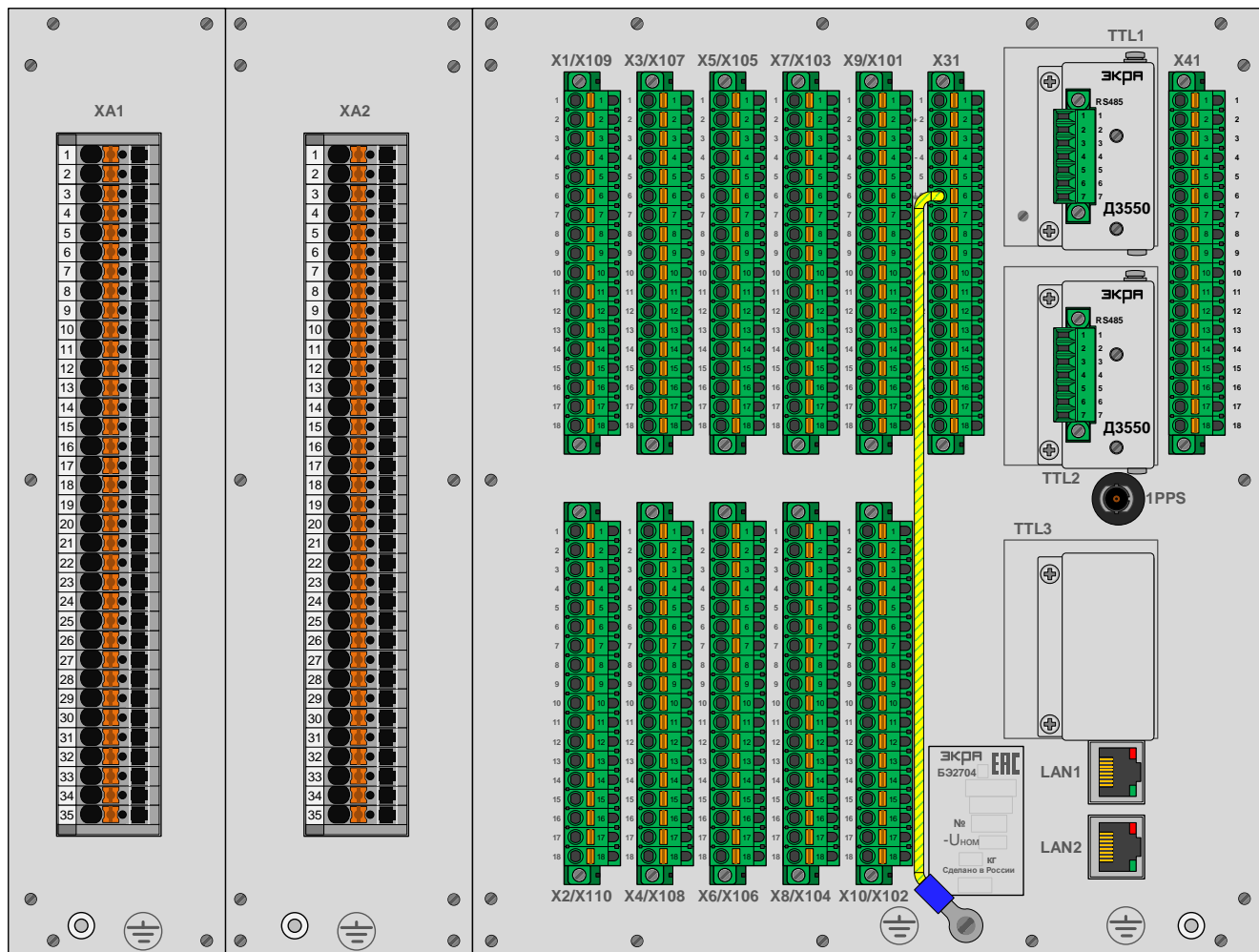
Рисунок 18 – Расположение элементов на задней панели терминала защиты БЭ2704 308
