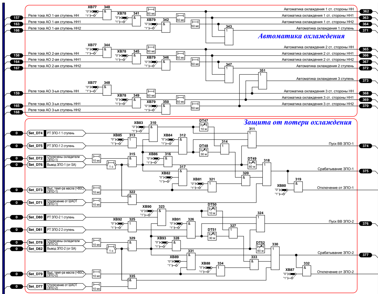
Рисунок 3 – Функциональная логическая схема блока логики автоматки охлаждения
