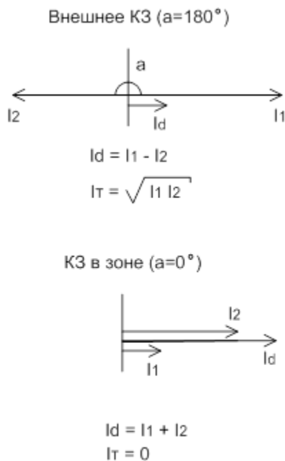
Рисунок 12 – Определение дифференциального и тормозного токов ДЗО НН
