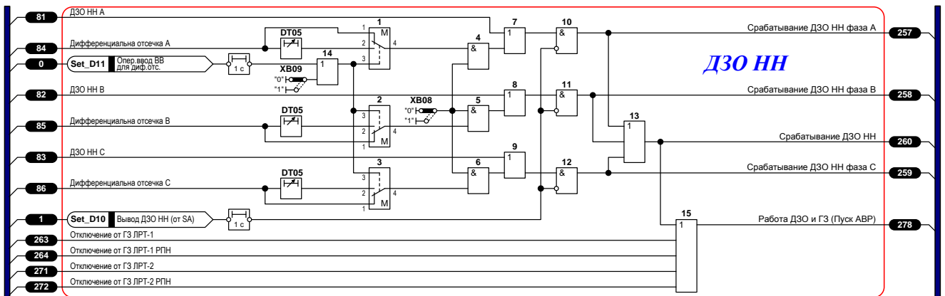
Рисунок 1 – Функциональная логическая схема блока логики ДЗО НН
