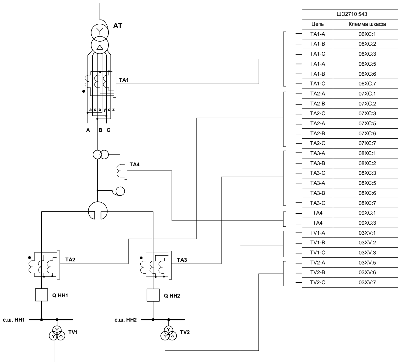
Рисунок 10 - Схема подключения ШЭ2710 543 к цепям переменного тока и напряжения
